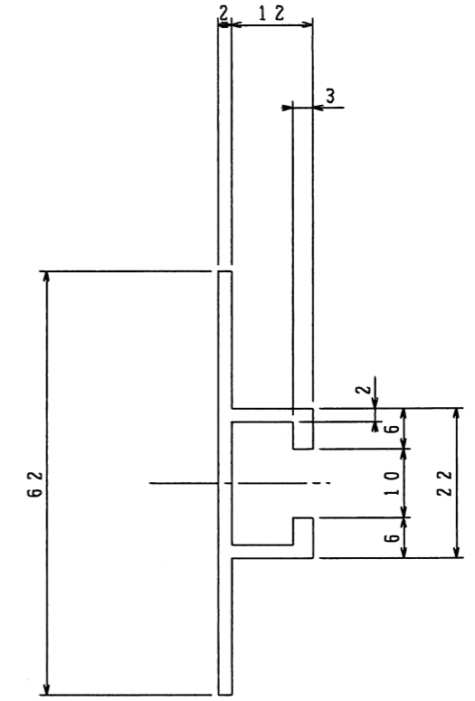
補強板詳細
