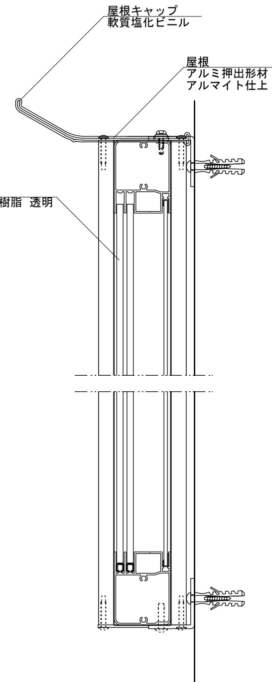
【側断面図 S=1:3】
