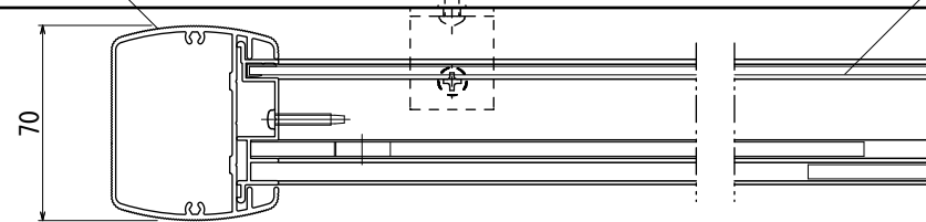
【平面図 S=1:3】
