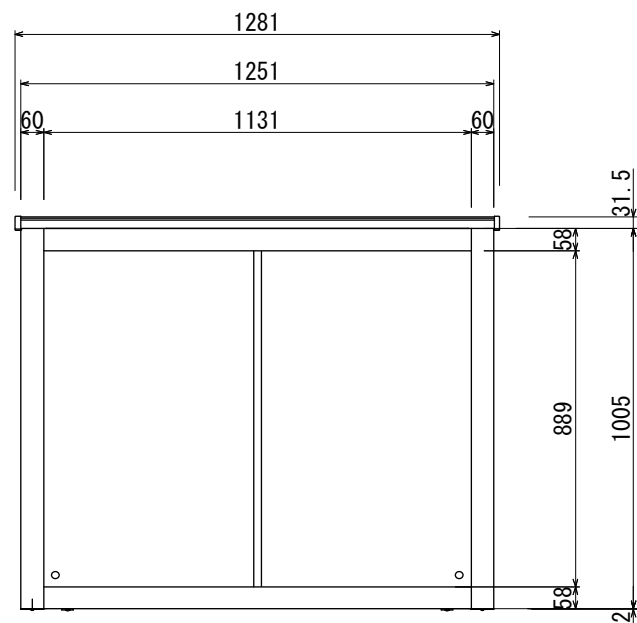
【正面図 S=1:20】
